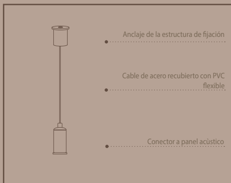
Colgante tensor de anclaje a losa
