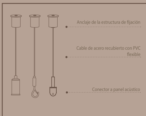
Colgantes tensor de anclaje a losa
